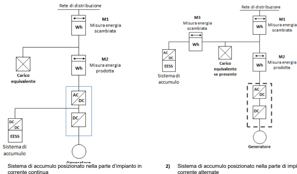
Figura 2: Schemi d'impianto realizzabili con REACT 2
